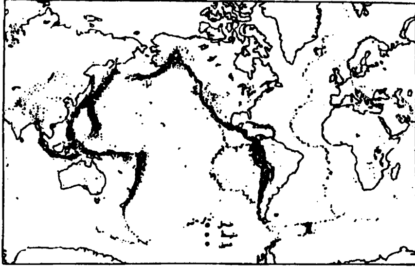
توزيع الزلازل: ضحلة، ومتوسطة، وعميقة المركز
